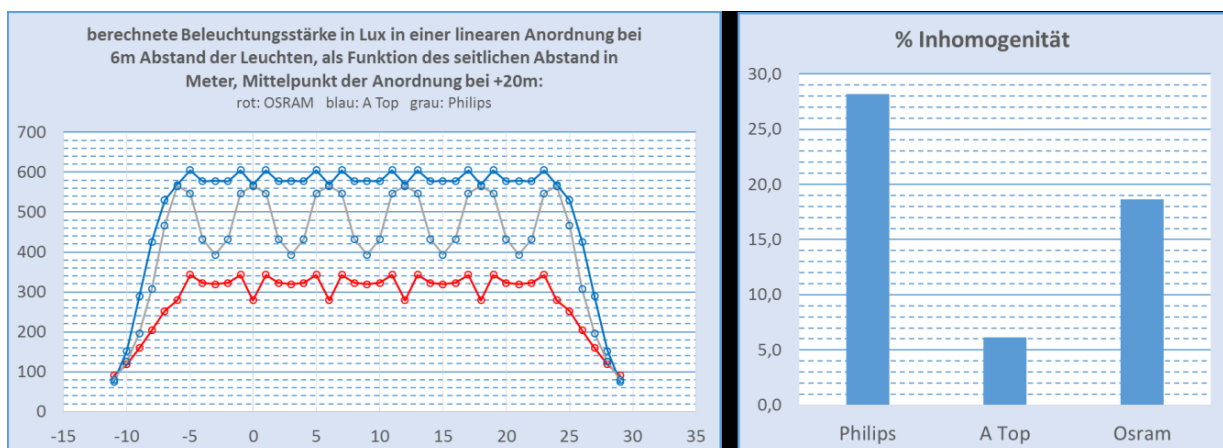
Rys. 5 Obliczone natężenie oświetlenia w luksach dla 3 produktów testowych rozmieszczonych w siatce liniowej w odległości 6 m, na wysokości 5,14 m, zainstalowanych w standardowej oprawie dla lamp HQL (po lewej), czerwony: Osram, niebieski: ATop, szary: Philips. Po prawej porównanie niejednorodności oświetlenia (bez obszarów brzegowych).
