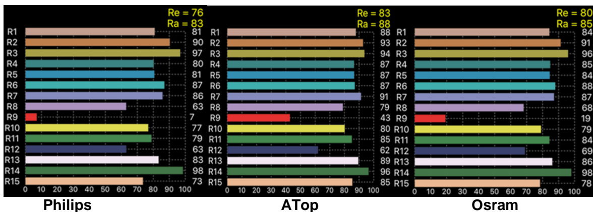
Rys. 9 Porównanie współczynnika oddawania barw dla 3 produktów testowych w odniesieniu do standardowego konwencjonalnego źródła światła ze 100% współczynnikiem odwzorowania wszystkich 14 standardowych barw. Zauważalna jest największa różnica dla parametru R9 (kolor czerwony). Ze wszystkich 3 testowanych produktów reemisja barw dla tego koloru jest najlepiej reprezentowana przez model ATop i jest ona 2 a nawet 3 razy wyższa niż w pozostałych dwóch testowanych produktach.
